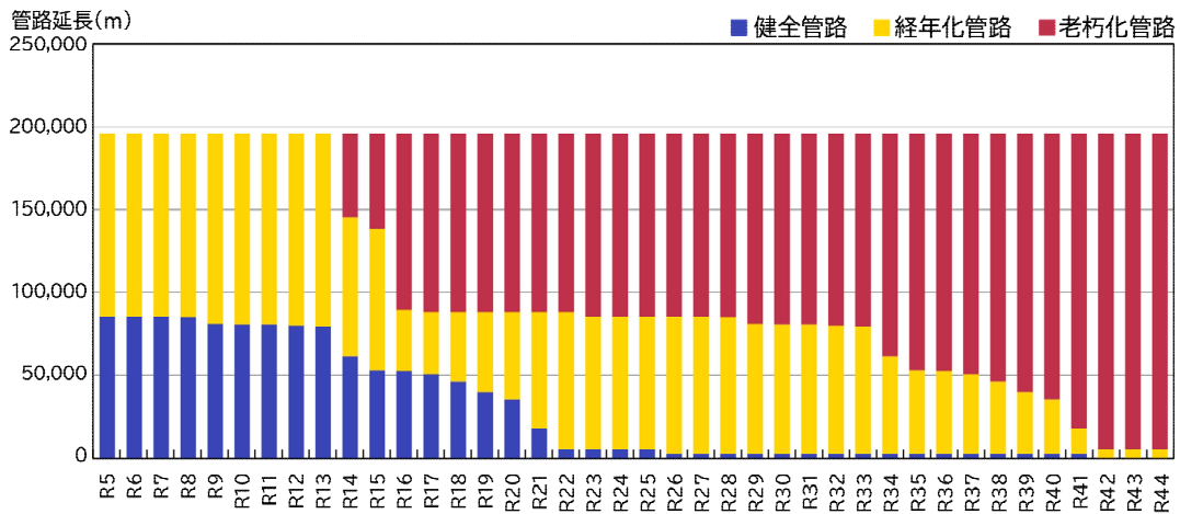
図 2.5 管路の健全度推移（m）
