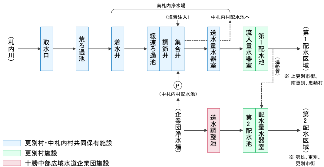
図 1.3 施設フロー
