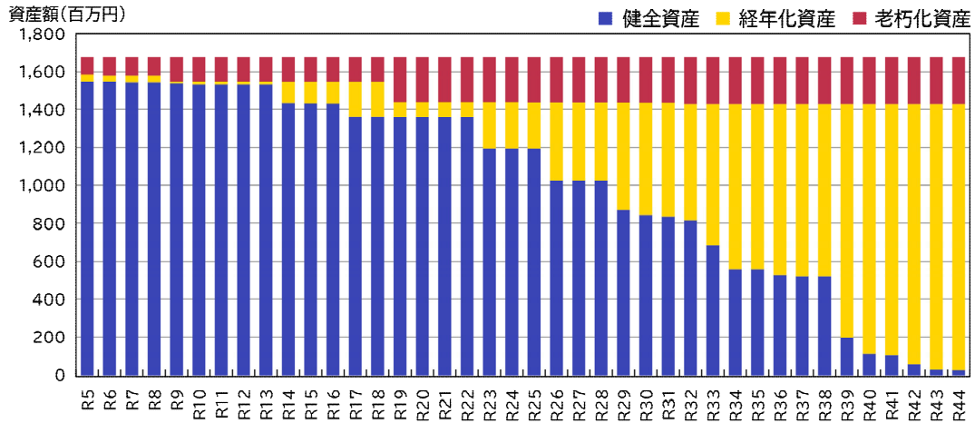
図 2.4 施設・設備の健全度推移（単位：百万円）
