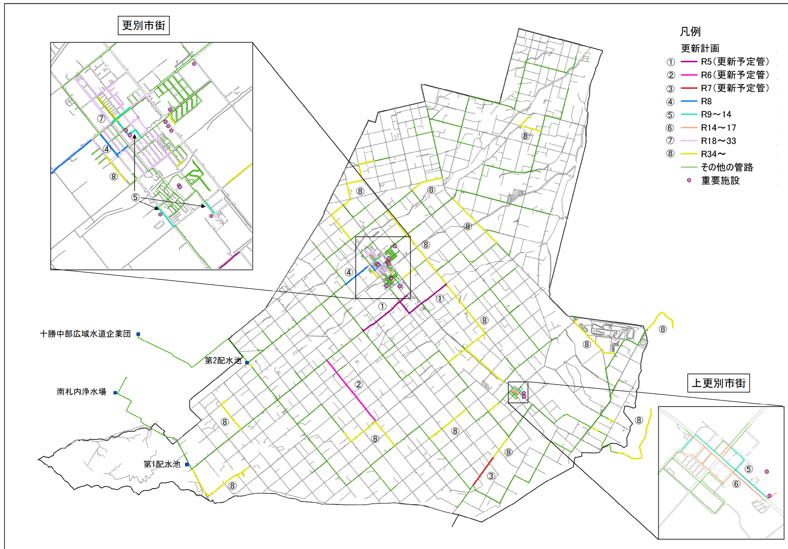
図 4.11 管路更新計画
