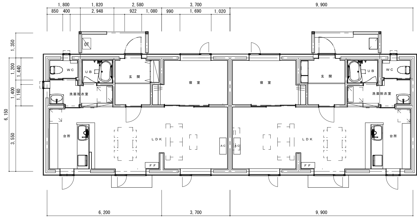
定住化促進住宅新栄 平面図
